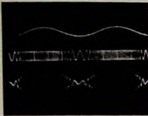
Afb. 14. AM en FM gemoduleerd. Realisatie: 1-sweep + niveau 2-gesweepde VCO 3-analoge vermenigvuldiger
